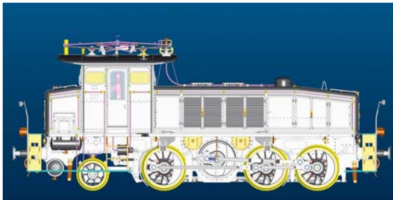
Konstruktionszeichnung
